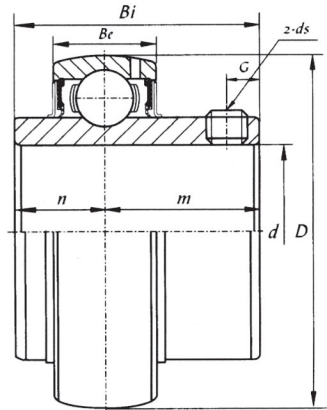
UCX00 (medium-duty)
