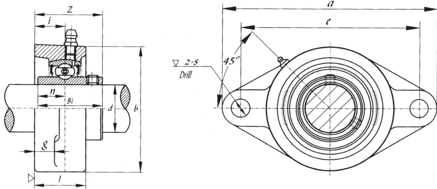
UCFLX00 (medium-duty)
