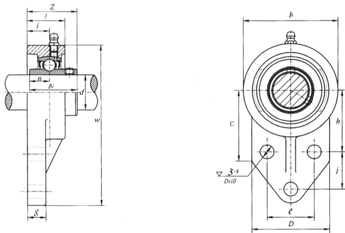
UCFB 200 (normal-duty)
