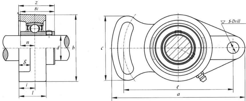
UCFA 200 (normal-duty)
