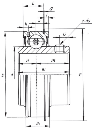
SER 200 (normal-duty)
