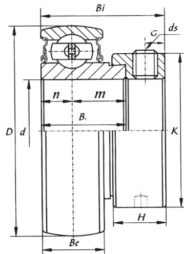
SA 200 (light-duty) Spherical O.D.
