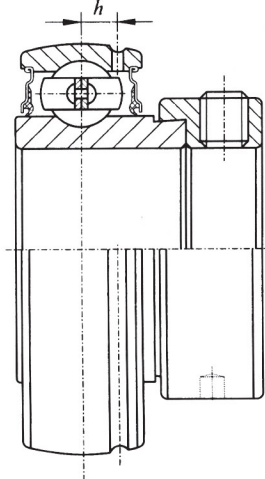
SA 200G Relubricatable type
