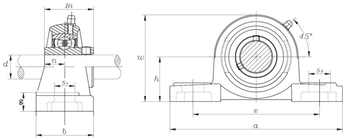
UCPX00 (medium-duty)
