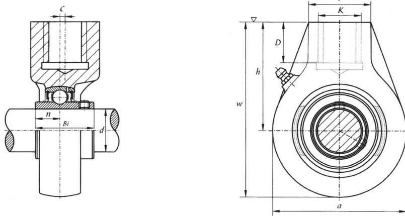
UCHA 200 (normal-duty)
