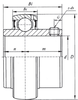
UC 200 (normal-duty)
