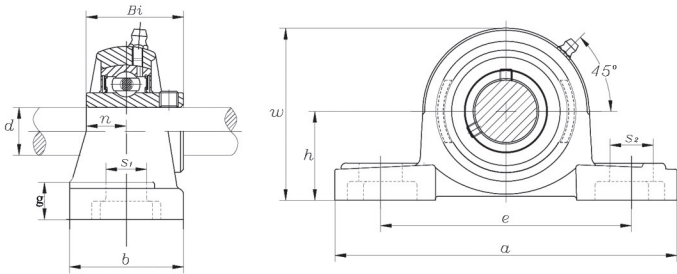
UCP 200 (normal-duty)
