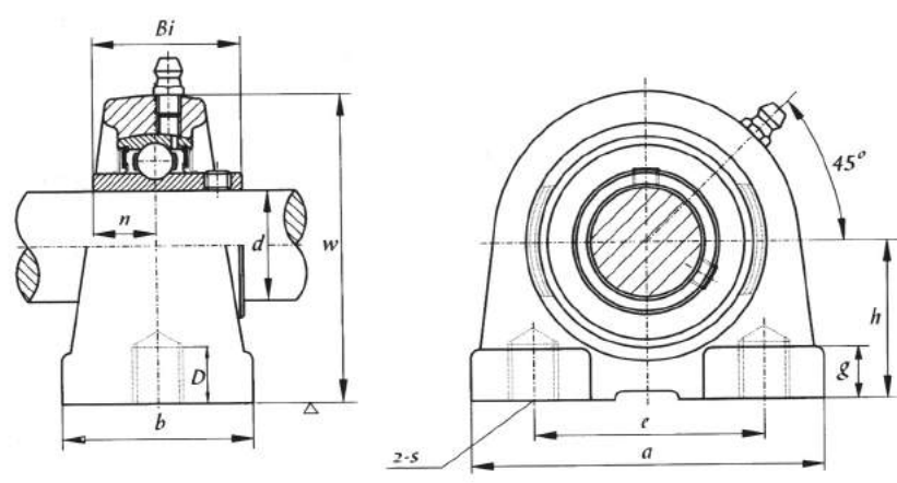
UCPA 200 (normal-duty)
