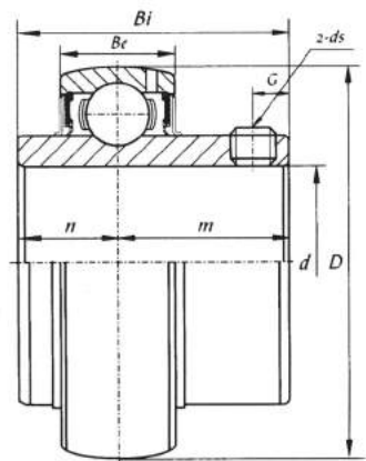
UC 200 (normal-duty)
