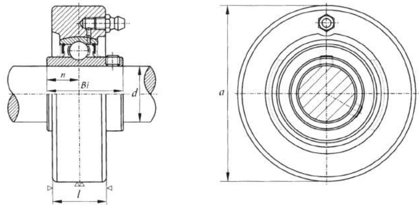
UCC 200 (normal-duty)
